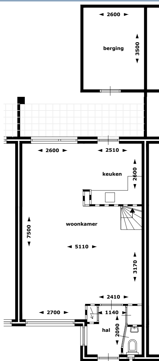
begane grond
