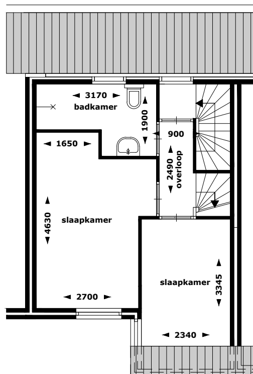
eerste verdieping
